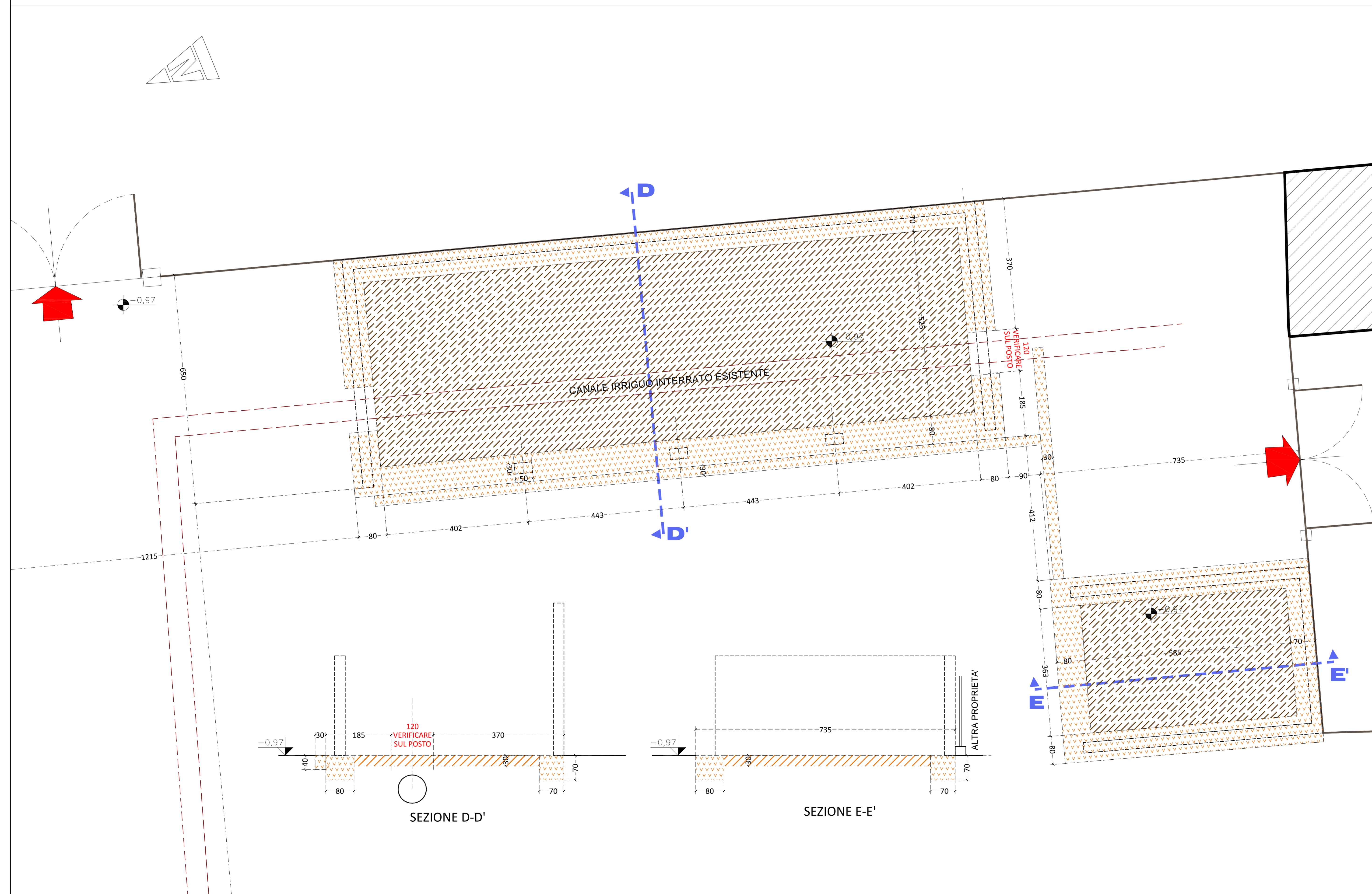
PLANIMETRIA AREA AUTORIMESSE
