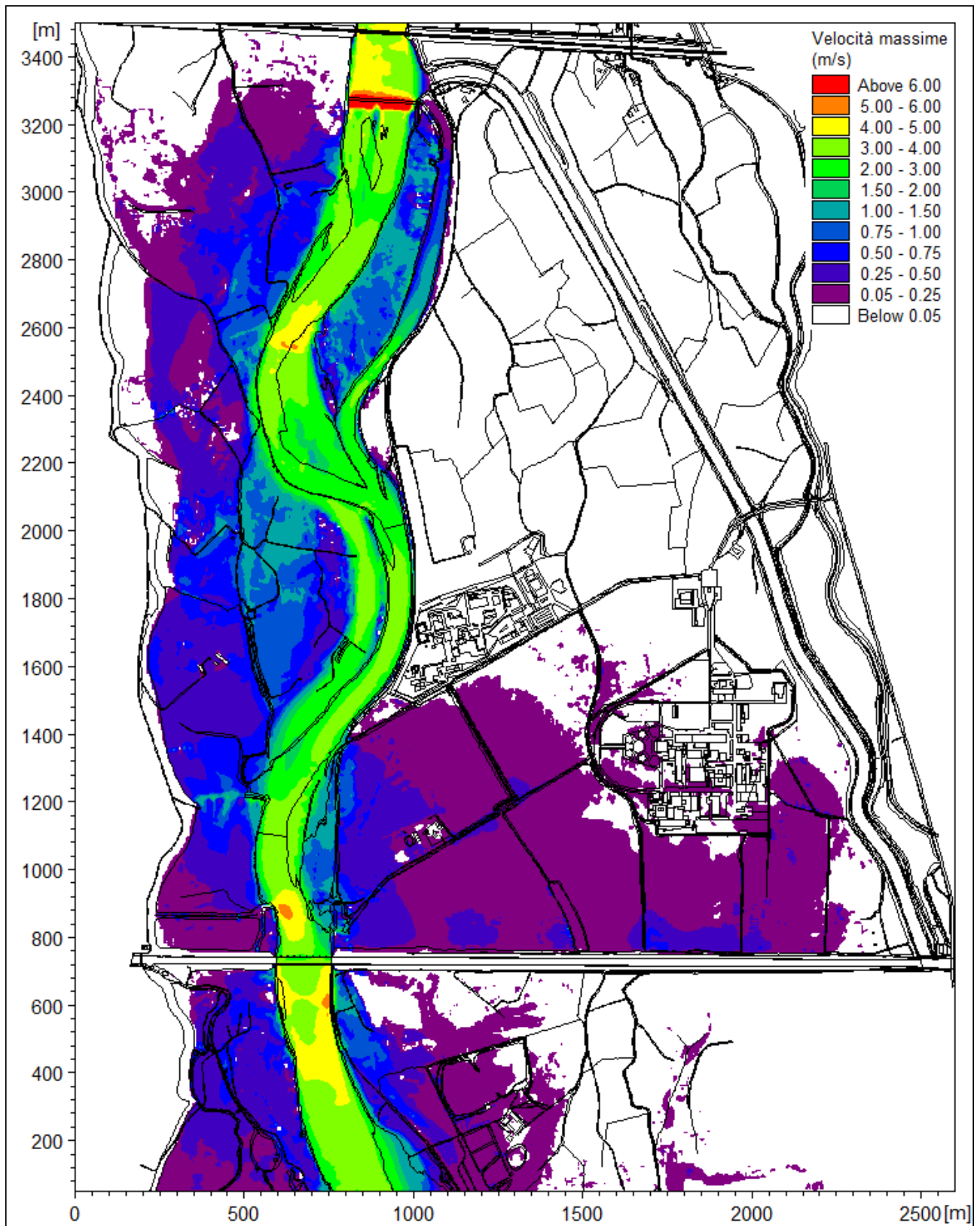
Figura 21 - Scenario con tempo di ritorno 200 anni "senza barriere". Mappa delle velocità massime.
