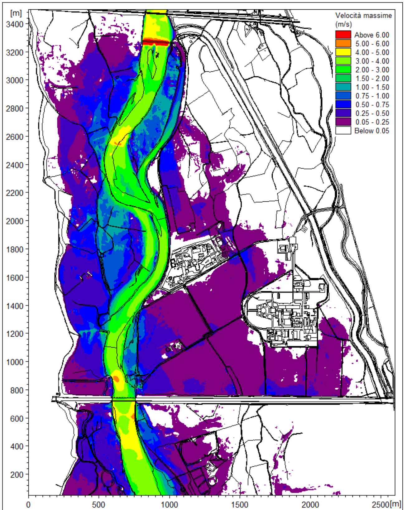
Figura 19 - Scenario con tempo di ritorno 200 anni con rota arginale. Mappa delle velocità massime.
